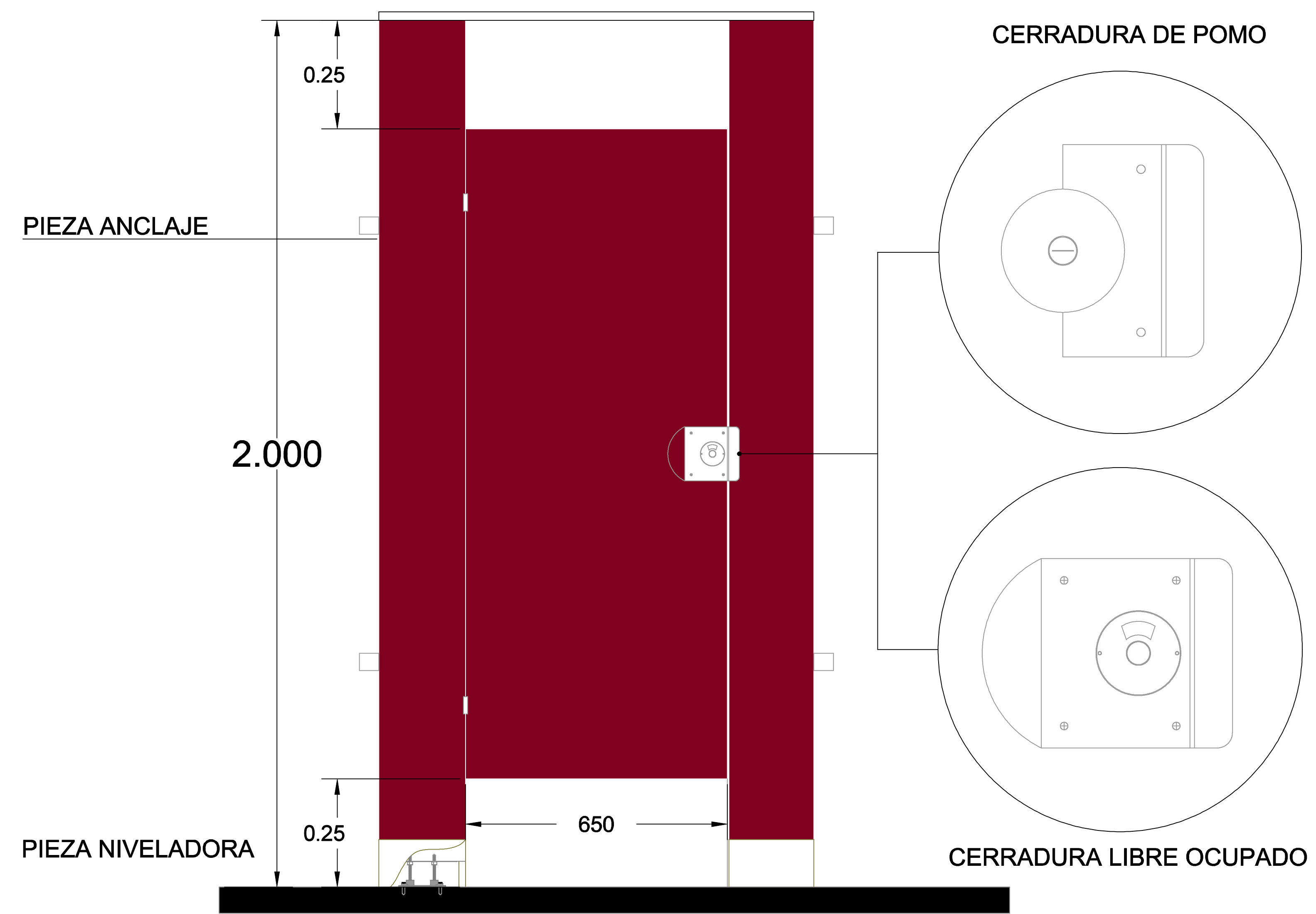
FRENTE
